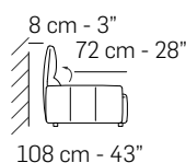
parete // wall
